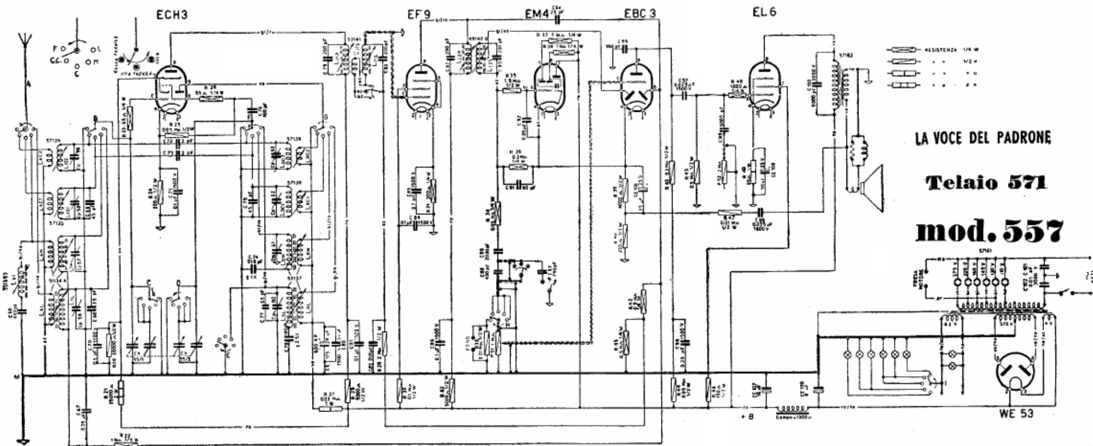
LA VOCE DEL PADRONE. — Mod. « 557 » radiogrammofono. — Produzione: 1940-1941. — Media frequenza: 465 kHz. — Gamme: c.c. (14,5-27 m), c. (23-56 m), m. (192-580 m), l. (860-2000 m). — Consumo: 60 watt circa. Potenza d'uscita: 6 watt.
